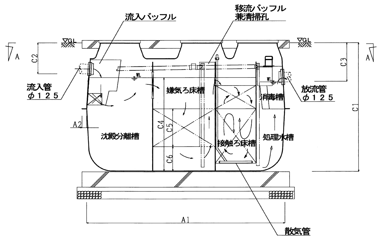
B-B断面図
