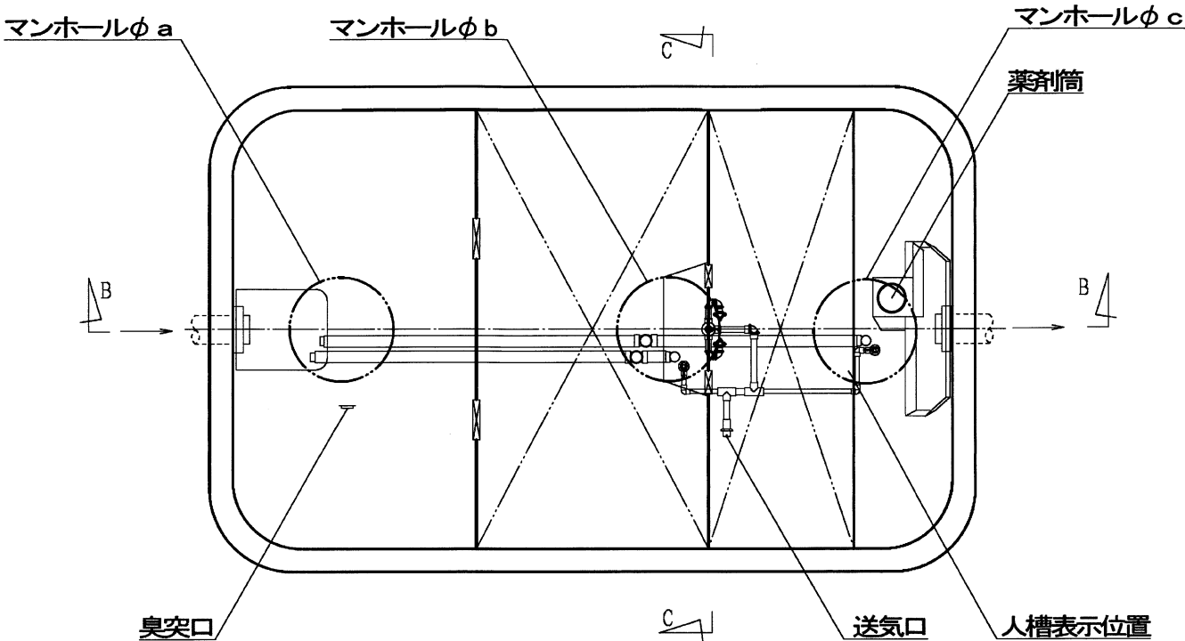
A-A断面図
