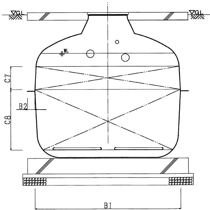
C-C断面図
