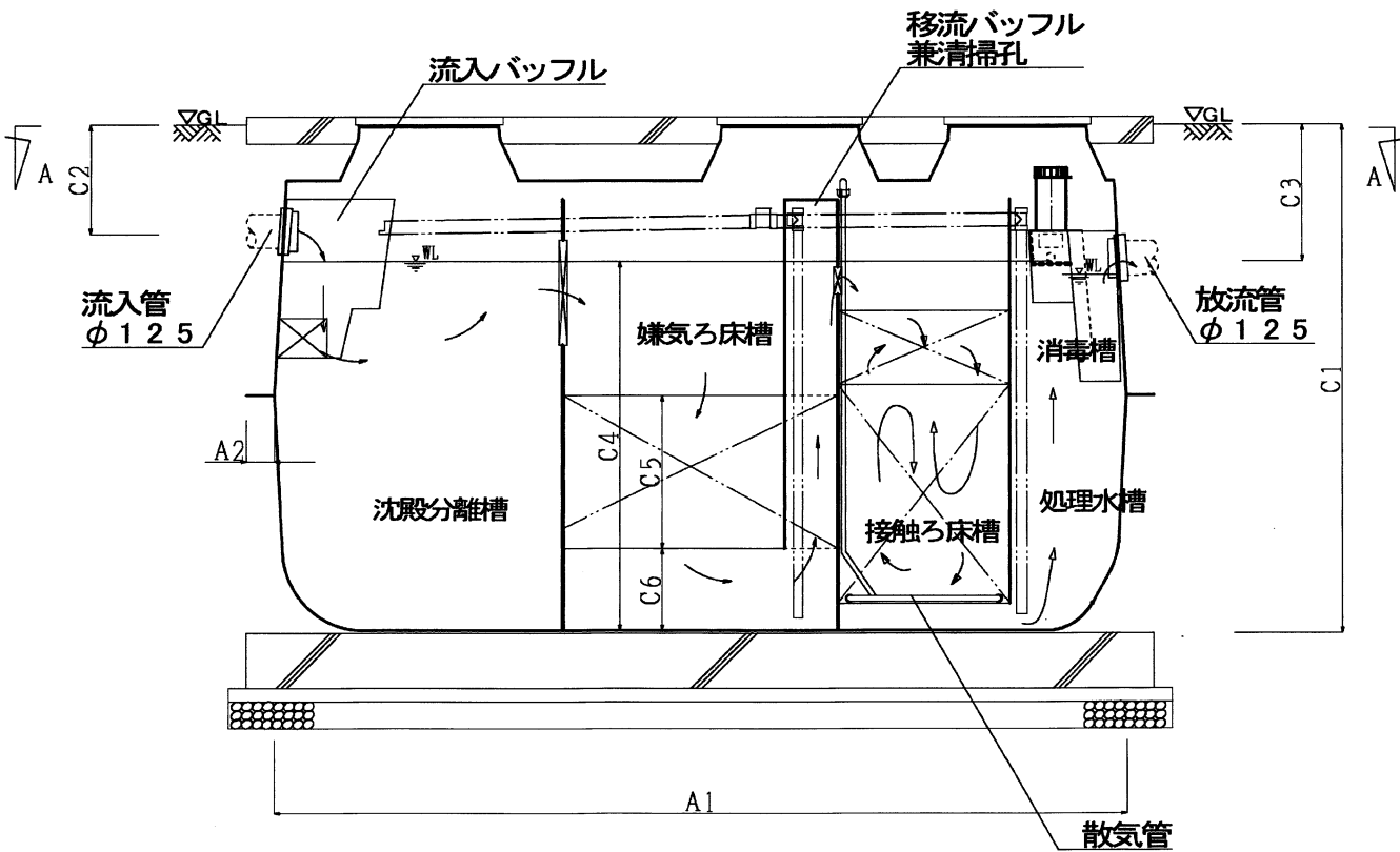
B-B断面図
