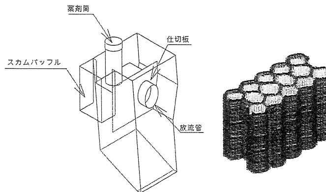
消毒槽立体図
