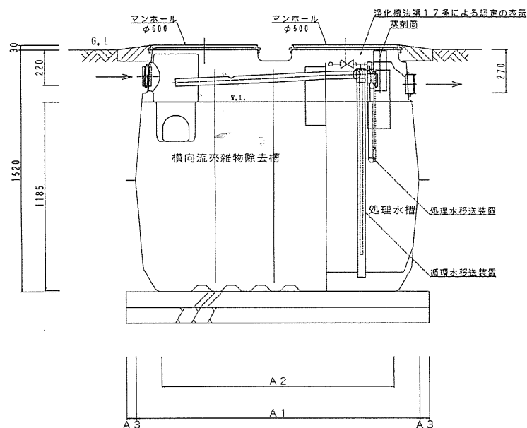
A-A断面図
